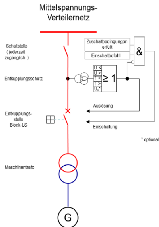
Abbildung 17: Netzanschluss an das Mittelspannungsnetz mit Netzentkuppungsschutz
