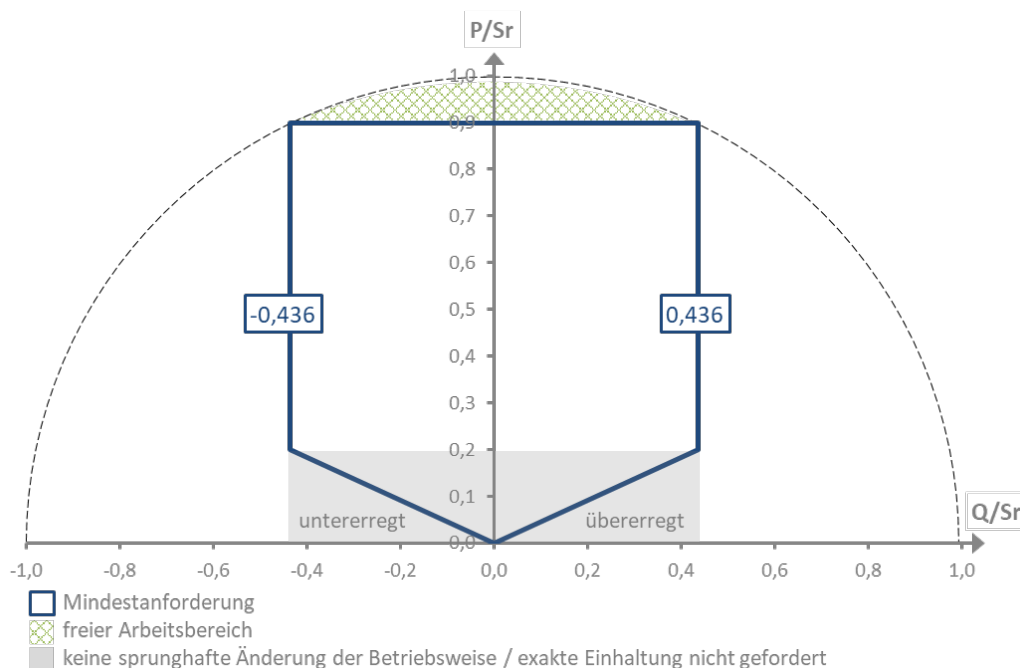
Abbildung 11: Blindleistungsbereich von Stromerzeugungsanlagen mit S_r > 3,68 kVA unterhalb der Nennscheinleistung
