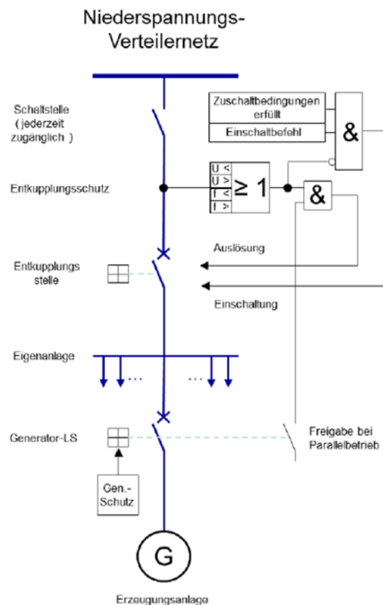
Abbildung 16: Netzanschluss am Niederspannungs-Verteilernetz mit zweiseitig versorgbarer Anlage des Netzbetreibers
