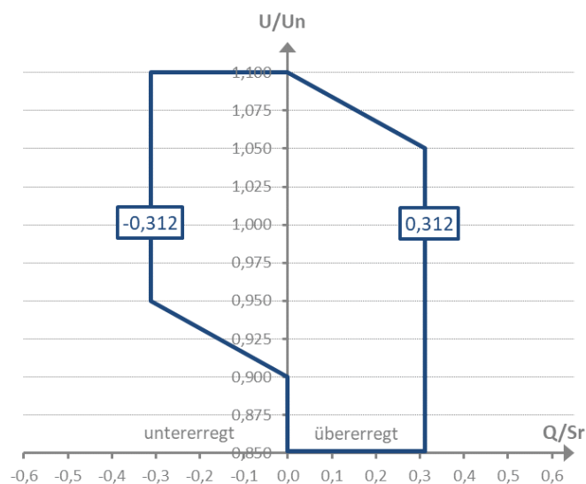
Abbildung 7: Blindleistungsbereich von Stromerzeugungsanlagen mit S_r \leq 3,68 \text{ kVA} (ohne Umrichter 15 ) bei Nennscheinleistung
